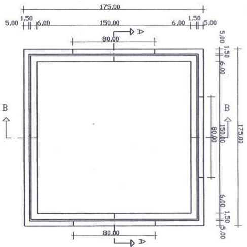
PIANTA POZZETTO
