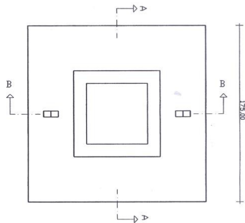
PIANTA COPERCHIO
