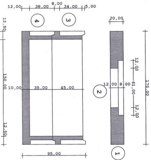
SEZIONE POZZETTO A-A
